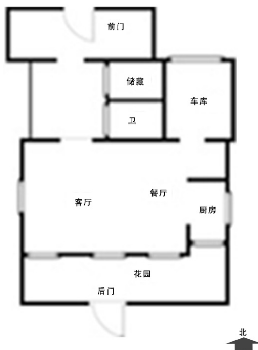
图5 联盟新城三期别墅某户一层平面图 (作者根据资料自绘)
