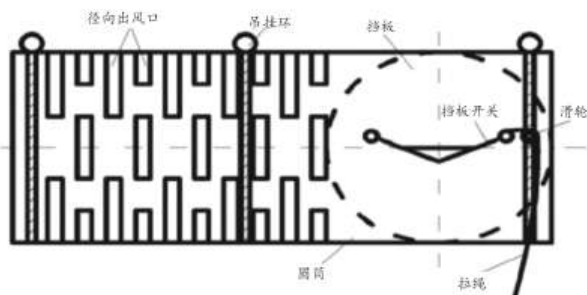
图2 附壁新型轻质风筒结构示意图
