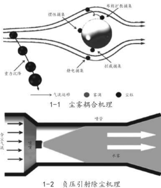
图1 机理示意图
