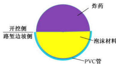
图3 新型同心不耦合护壁结构示意图
