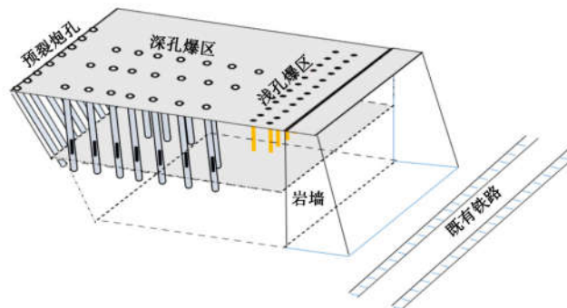
图2 不同的爆破方式分布示意
