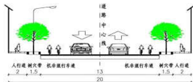
图1 市政道路设计断面示意图
