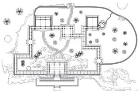
图2 绮望轩遗址复原平面图
