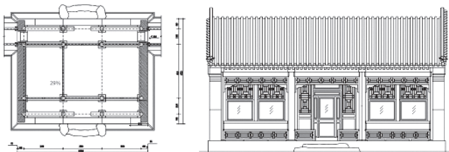
图1 绮望轩平面图及南立面图
