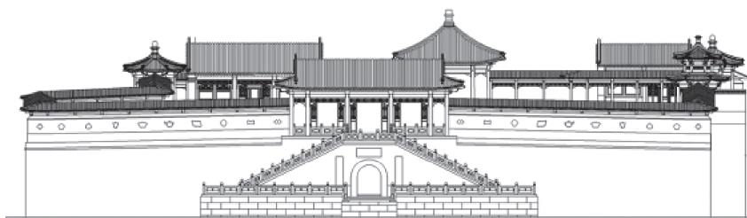
图3 绮望轩遗址复原北立面图
