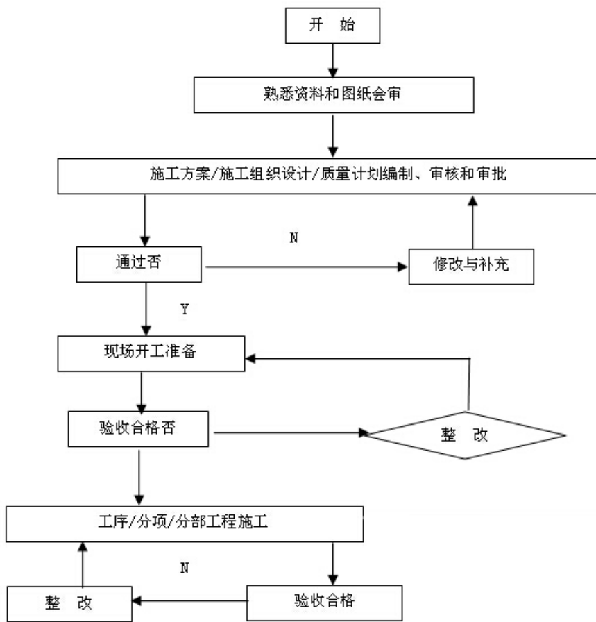
图1 建筑装饰施工流程图
