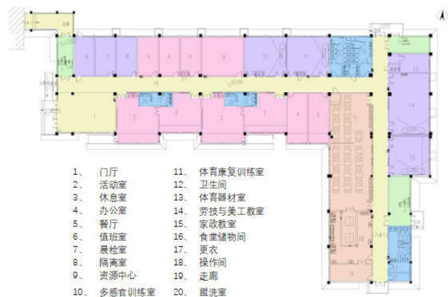
图2 一层平面图
