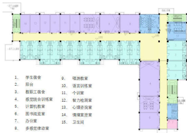
图3 二层平面图
